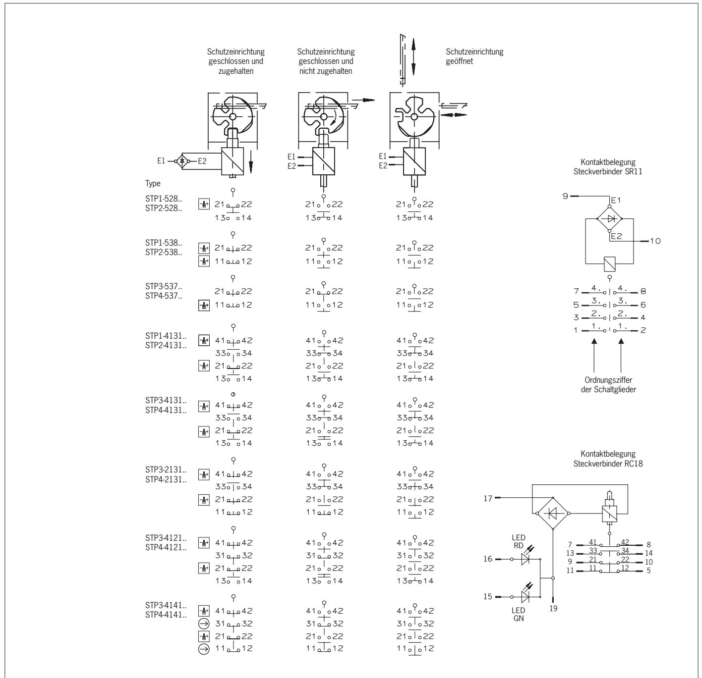
Bild 3: Schaltelemente und Schaltfunktionen
