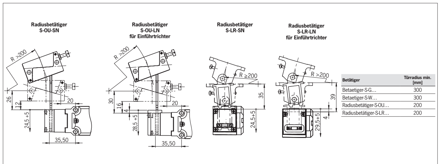
Bild 4: Minimale Türradien
