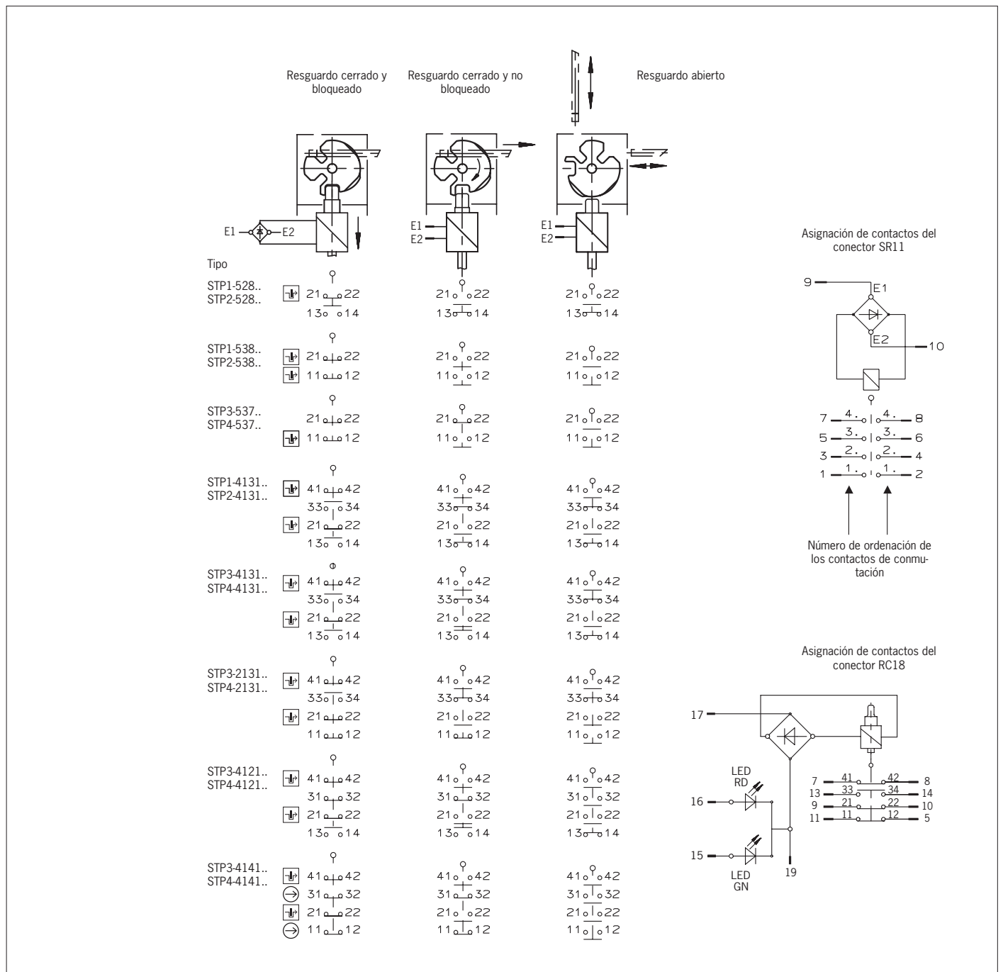
Fig. 3: Elementos interruptores y funciones de conmutación
