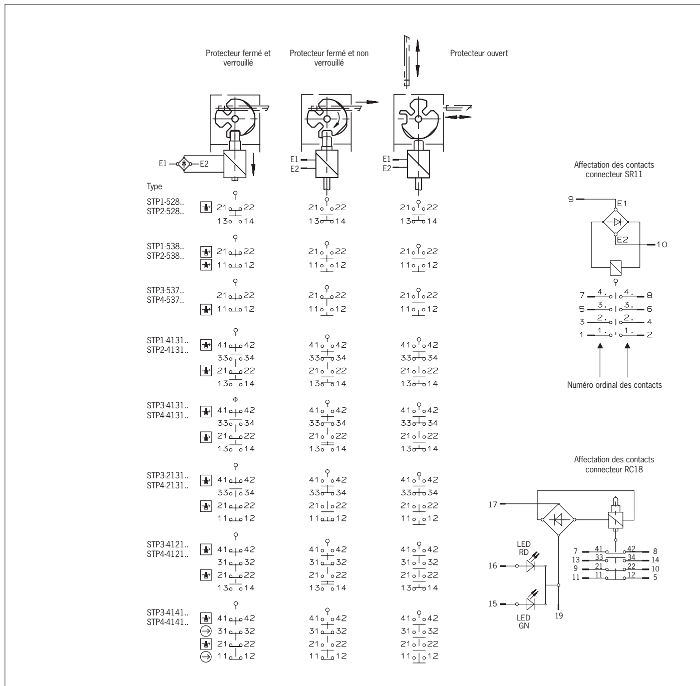
Fig. 3 : Éléments de commutation et fonctions de commutation
