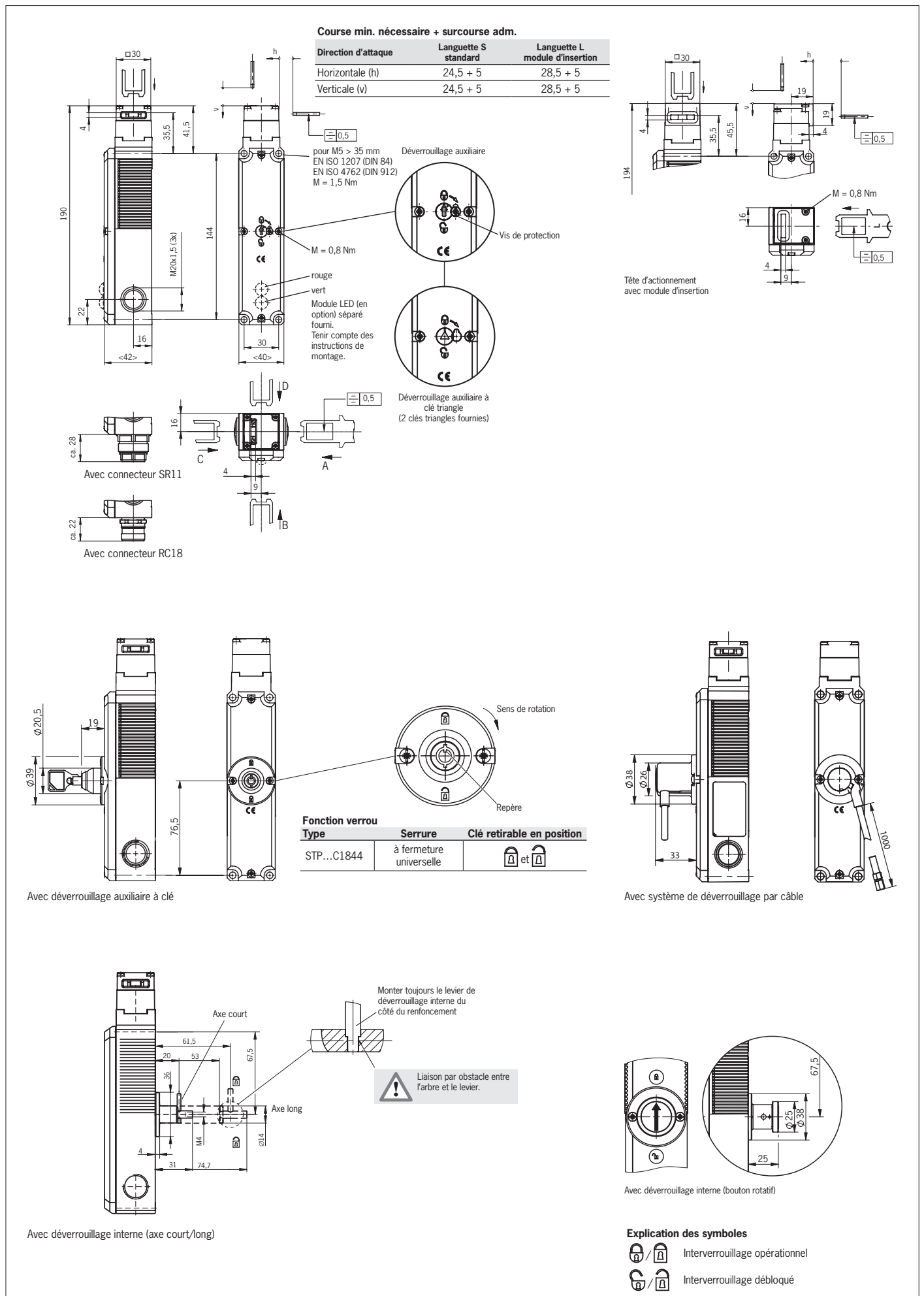
Fig. 2 : Dimensions STP... sans module d'insertion et STP... avec module d'insertion
