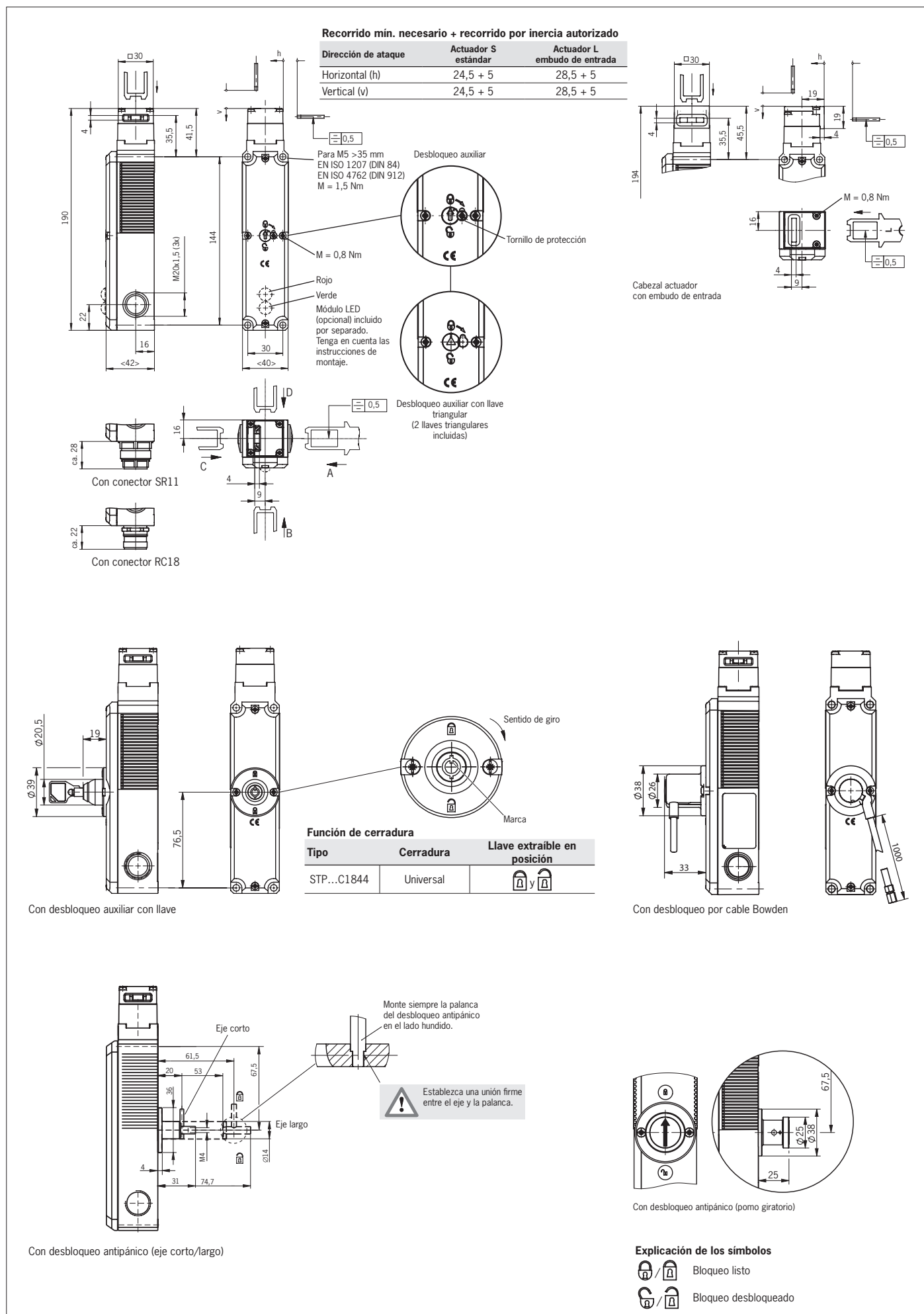
Fig. 2: Plano de dimensiones STP... sin embudo de entrada y STP... con embudo de entrada
